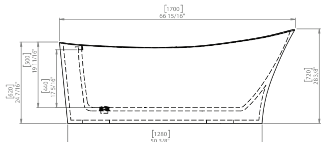
FRONT VIEW VUE DE FACE
