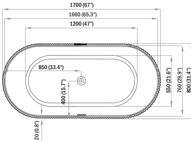
TOP VIEW -VUE DE DESSUS
