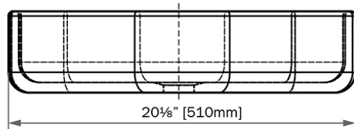
FRONT VIEW - VUE DE FACE
