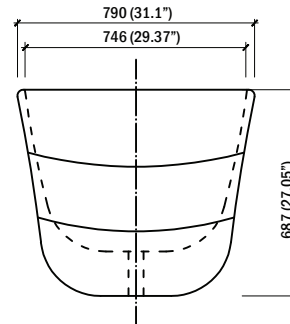
SIDE VIEW VUE DE CÔTÉ
