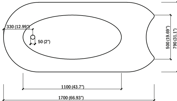
TOP VIEW VUE DE DESSUS
