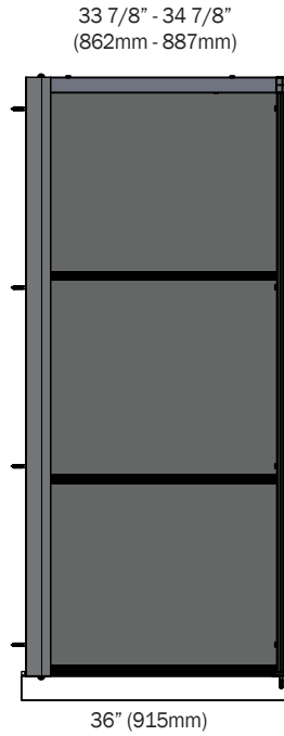
SIDE VIEW / VUE DE CÔTÉ
