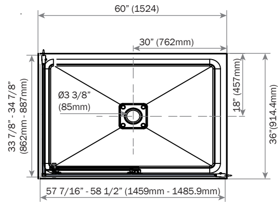
TOP VIEW / VUE DE DESSUS
