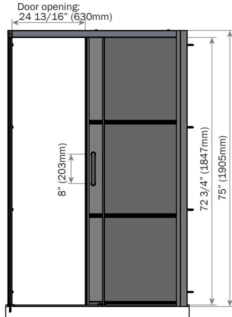
FRONT VIEW / VUE DE FACE
