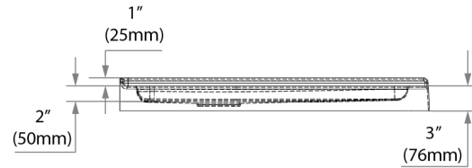
FRONT VIEW - VUE DE FACE
