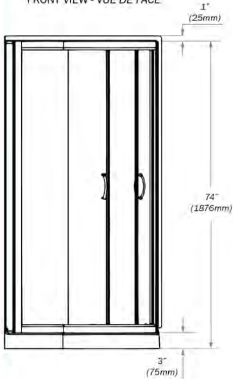
FRONT VIEW - VUE DE FACE
