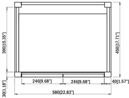
TOP VIEW / VUE DE DESSUS
