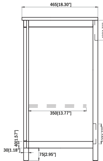
SIDE VIEW VUE DE CÔTÉ
