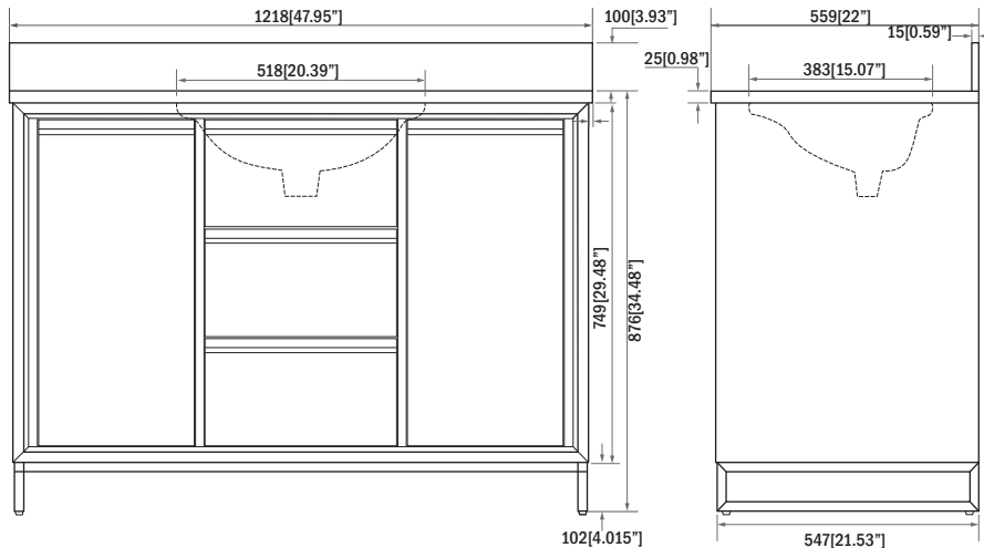
FRONT VIEW VUE DE FACE
