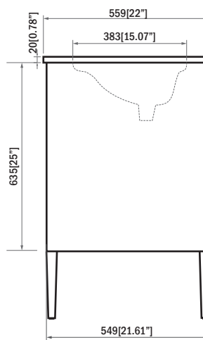
SIDE VIEW VUE DE CÔTÉ
