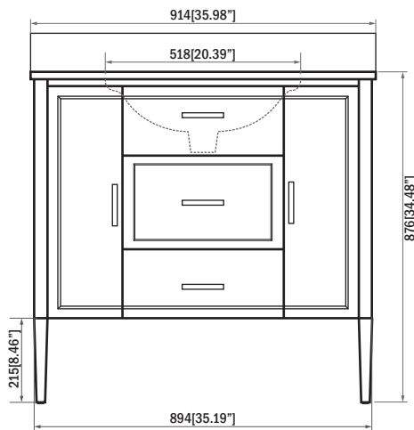
FRONT VIEW VUE DE FACE
