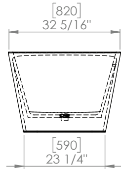
SIDE VIEW VUE DE CÔTÉ
