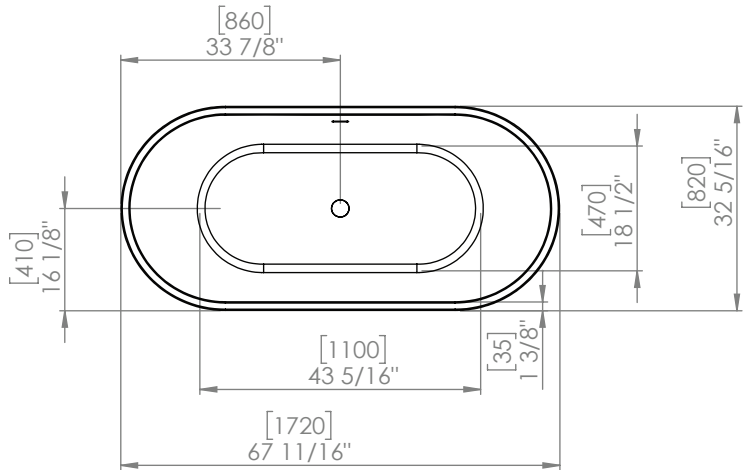
TOP VIEW VUE DE DESSUS
