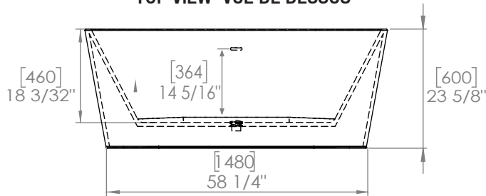
FRONT VIEW VUE DE FACE
